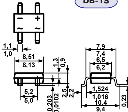
DB-1S
