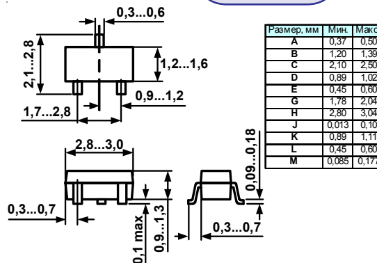
SOT-23
