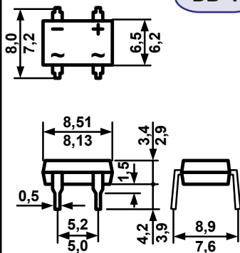
DB-1
