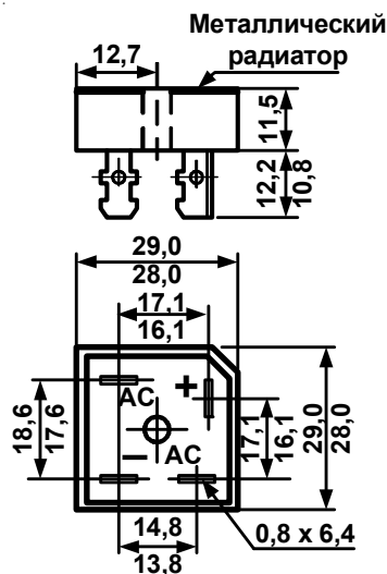
BR-25
