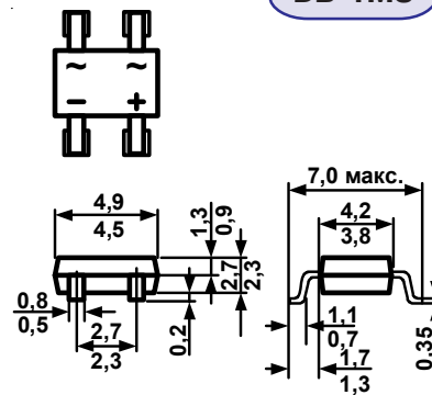
DB-1MS
